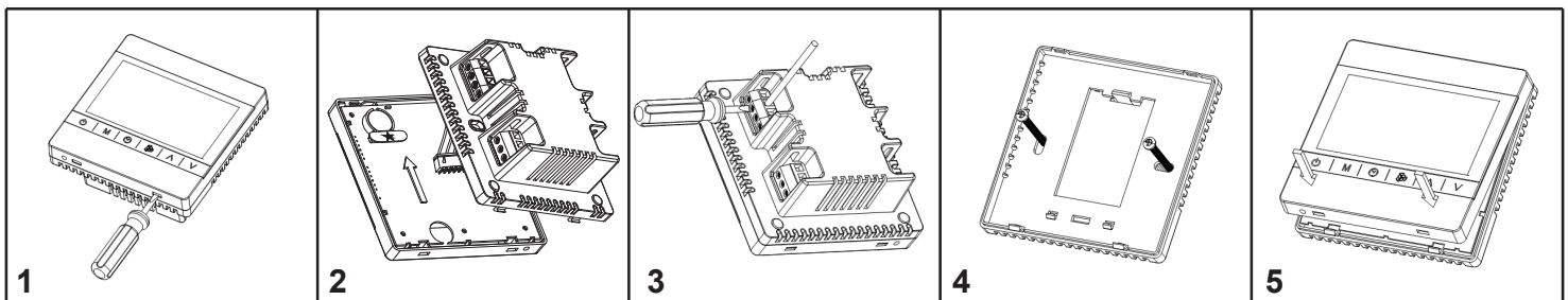
图 3: 安装说明图 Figure 3: Installation diagram
